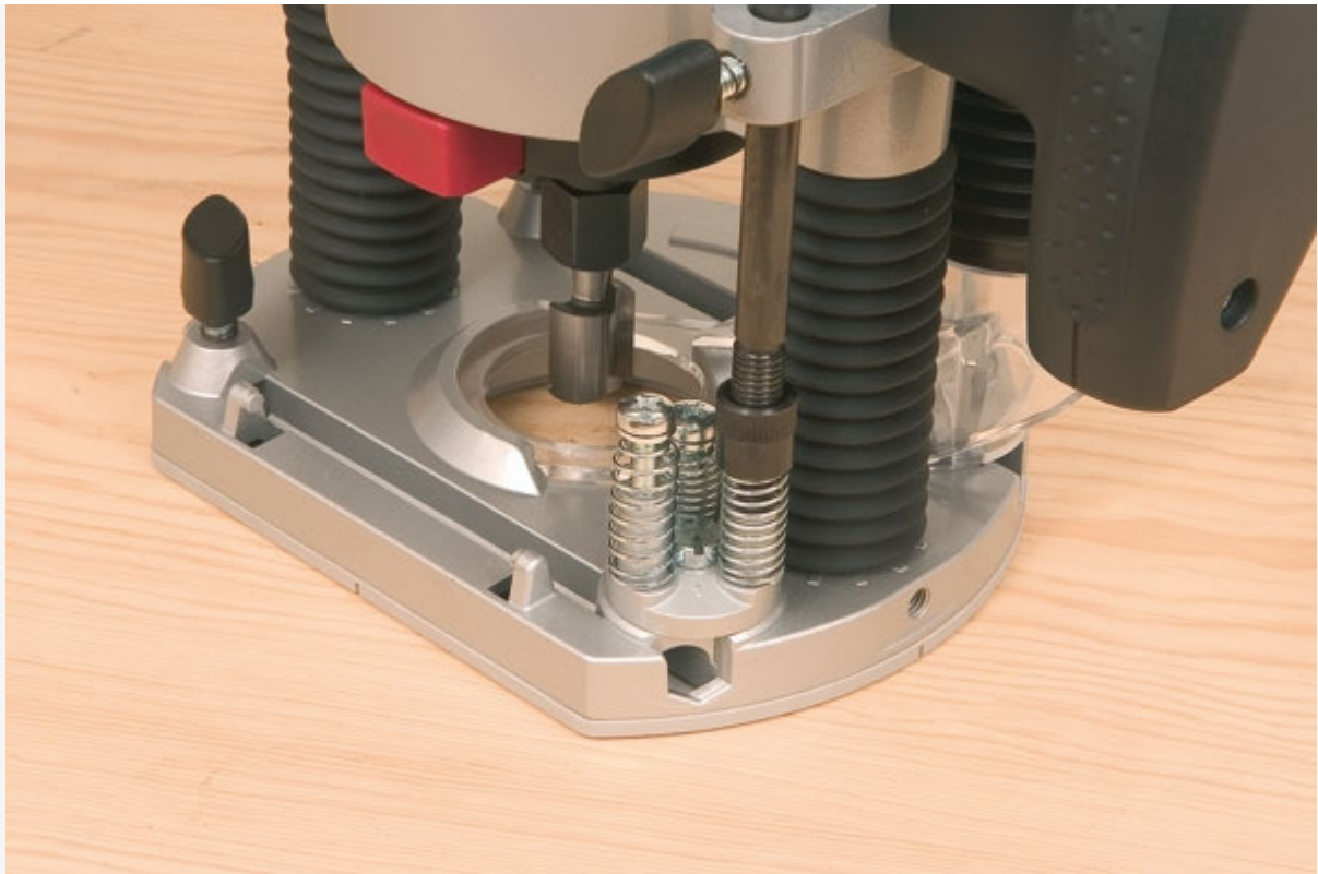
Réglage rapide de la profondeur de fraisage à 3 positions.
