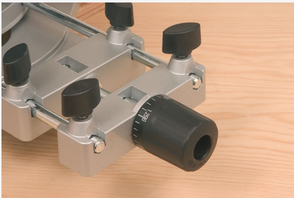
Équerre latérale à réglage micrométrique.
