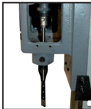
Système de mandrin pour fixation de la mèche Chuck tightened system to hold the chisel
