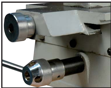
Chariotage latéral et longitudinal sur queue d'aronde Horizontal and lateral movement on dovetail
