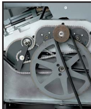
Entraînement des rouleaux par chaîne Entraînement moteur à double courroie Feeder drive chain Dual belt drive motor
